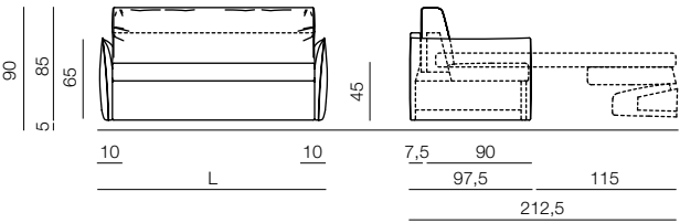
Variante seduta H.45 cm Seat variant H.45 cm Variante assise H.45 cm Variante Sitzfläche H.45 cm
