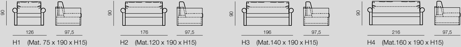
Seat variant H 50 cm and matt. H 15 cm / Variante assise h.50 cm et mat. h.15 cm / Variante Sitzfläche H. 50 cm und Mat. H. 15 cm
