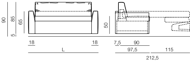
Variante seduta H.50 cm
