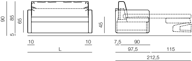
Variante seduta H.45 cm
